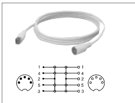
Cavo prolunga per tastiere Spine-presa 5 poli - Lunghezza 1,80 metri Ref. 3-072-405
